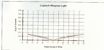
Zu geringer Kraftaufwand nötig, Auslenkung kaum spürbar.
